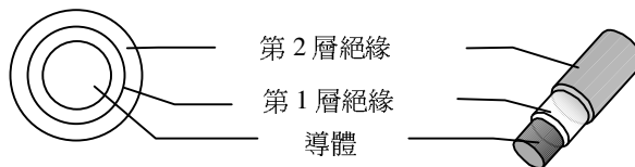
雙層絕緣線(DILW-F)構造
