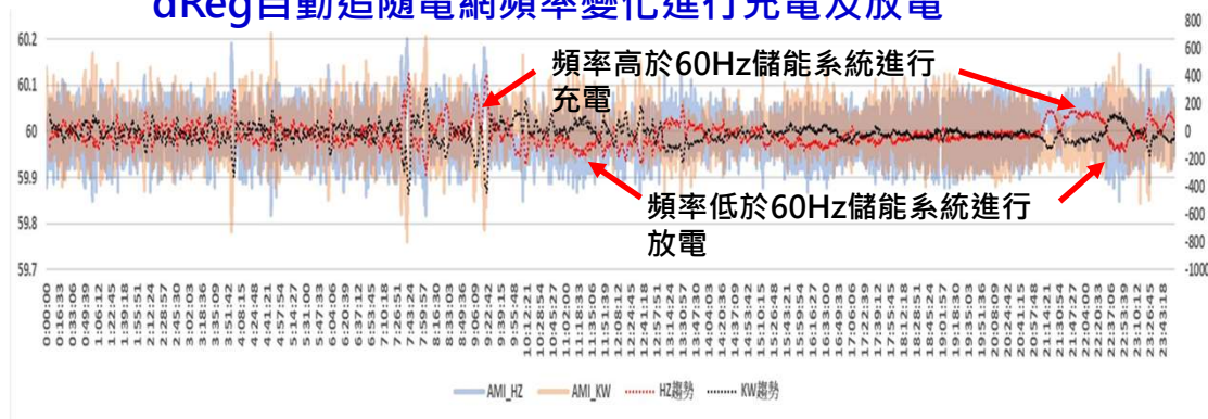
dReg自動追隨電網頻率變化進行充電及放電
