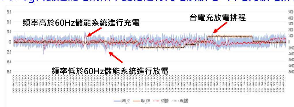
E-dReg自動追隨電網頻率變化進行充電及放電+台電充放電排程
