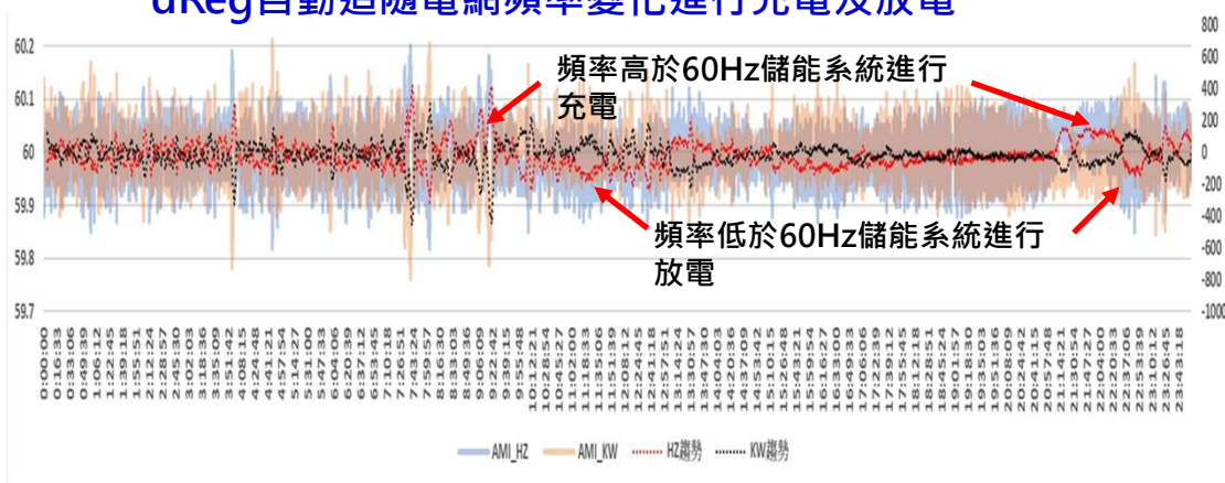
dReg自動追隨電網頻率變化進行充電及放電
